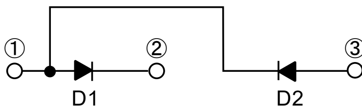
図 2. 回路図
