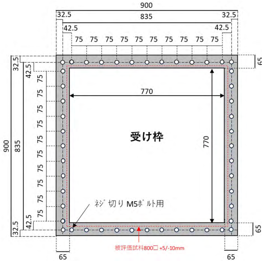
① 770□受け枠 t=5
