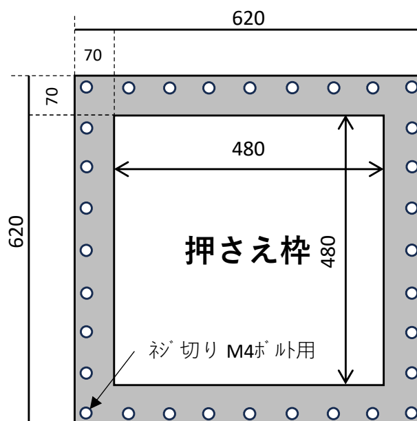
④ 480□押さえ枠 t=3
