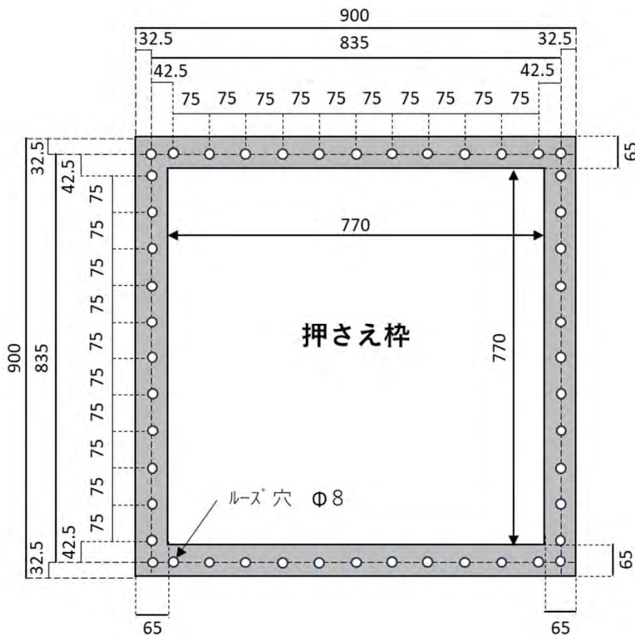
② 770□押さえ枠 t=3
