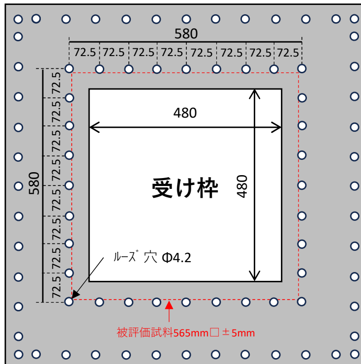
③ 770□→480□変換板(受け枠) t=3
